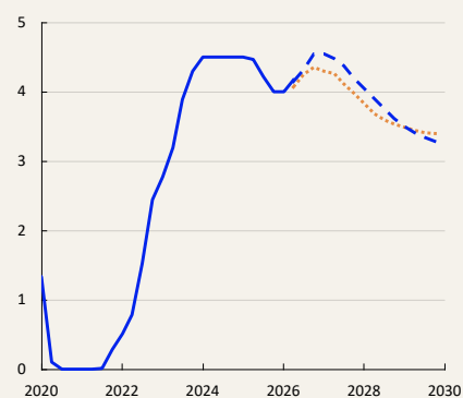
Styringsrente. Prosent
